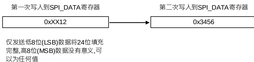
图 27-33 发送 0x123456
