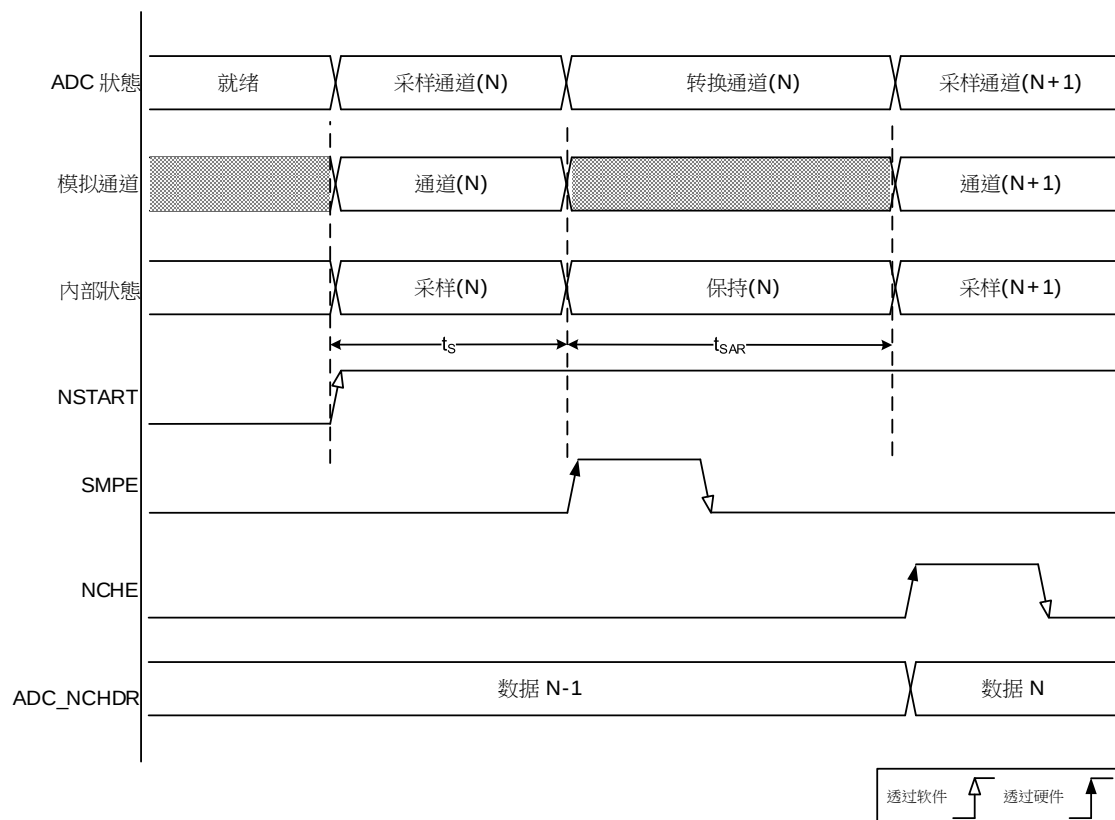
图 16-4ADC 标准转换
