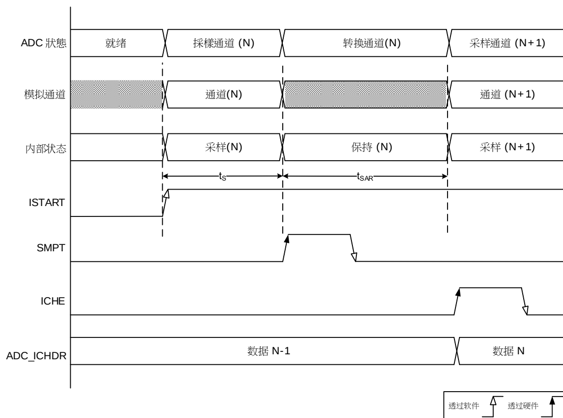
图 16-5 ADC 插入转换
