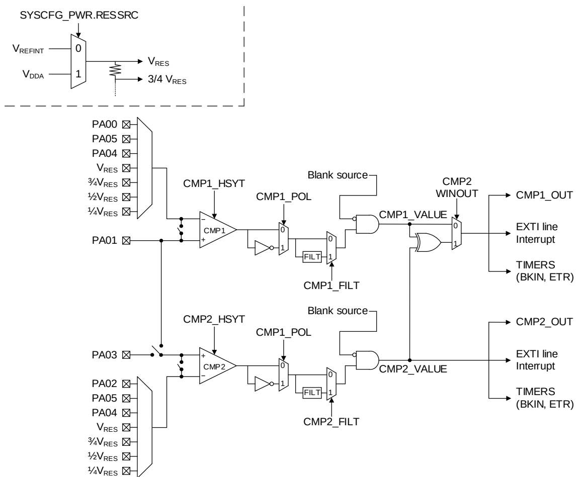
图 17-1 CMP 架构图
