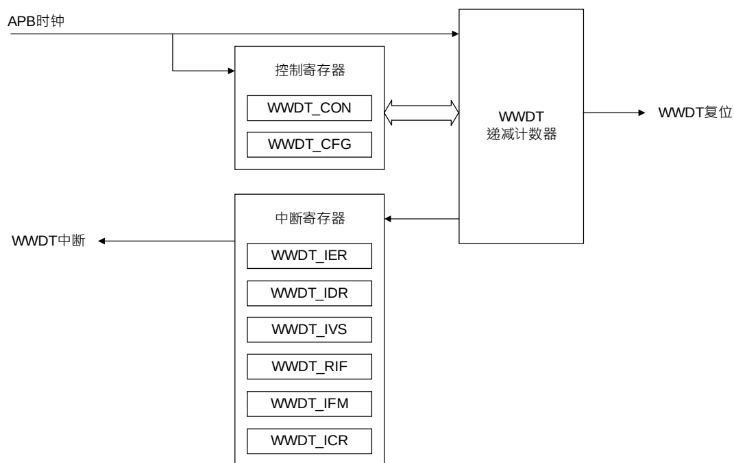
图 24-1WWDT 架构图
