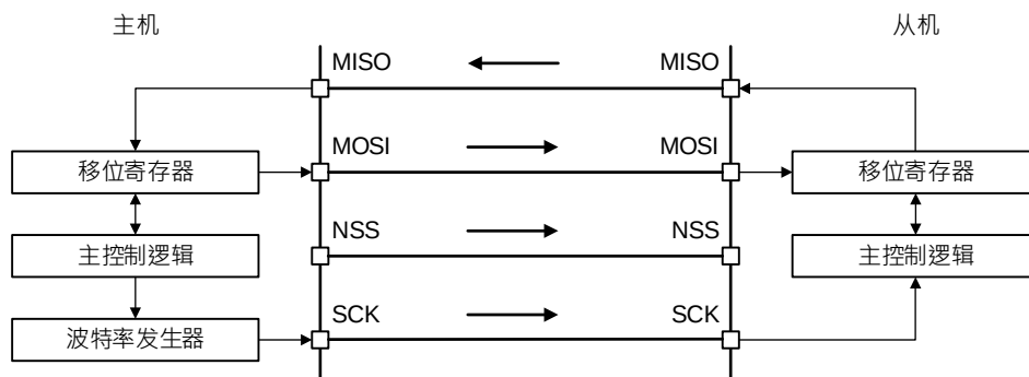
图 27-3 全双工通信
