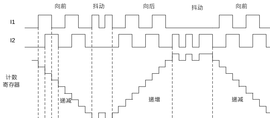
图 19-23 滤波后极性反相时编码器接口例子
