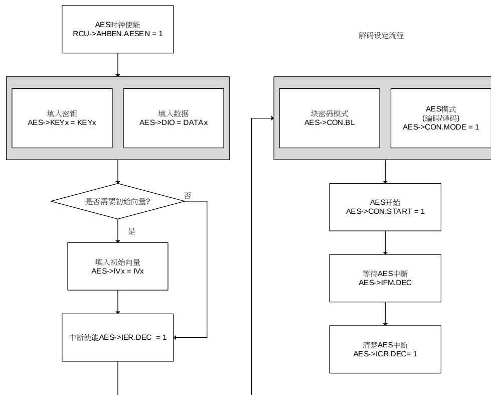
图 9-6 译码功能流程
